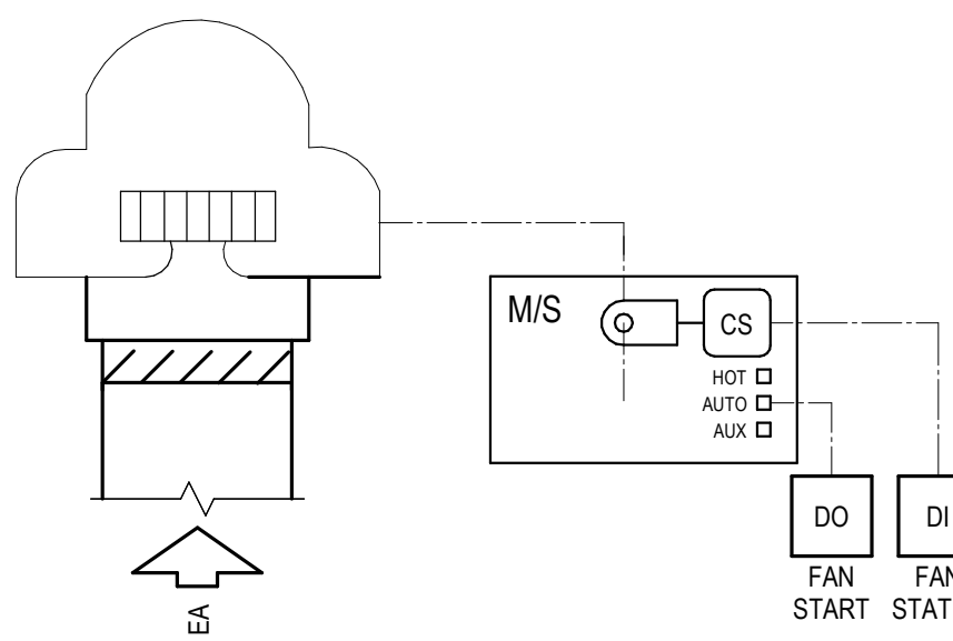
4 ROOF EXHAUST FAN
